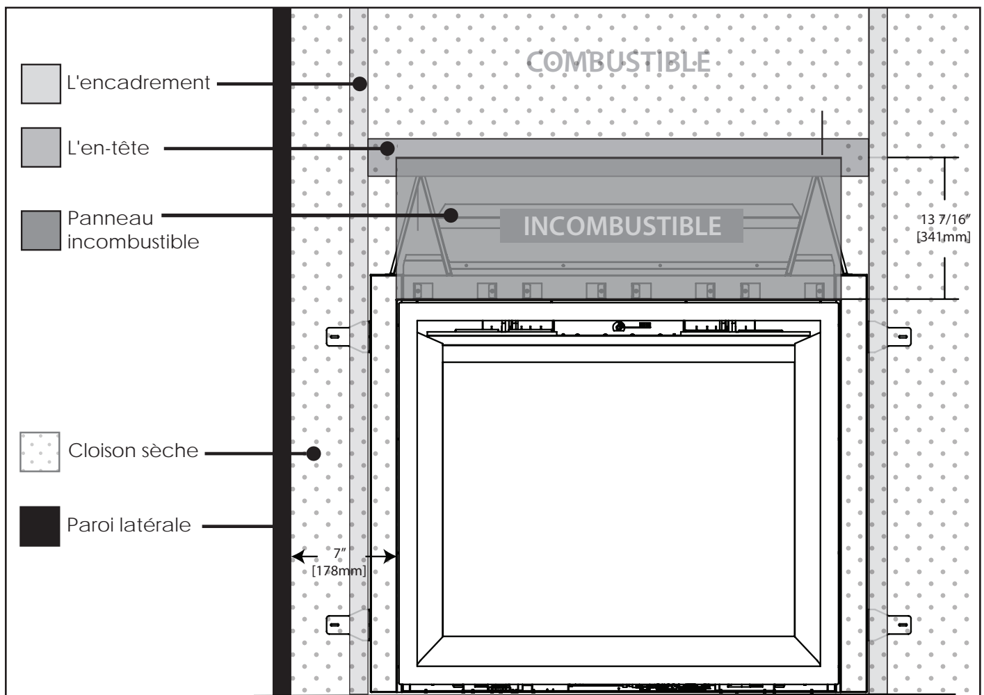
Figure 55. Disposition Face à Face Typique
