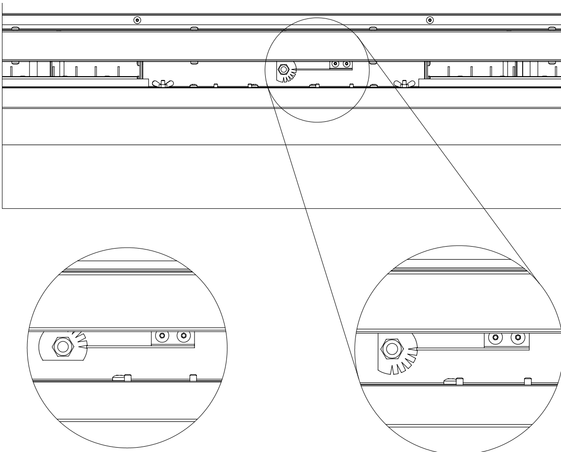
Figure 63. Réglage du Restricteur 1
