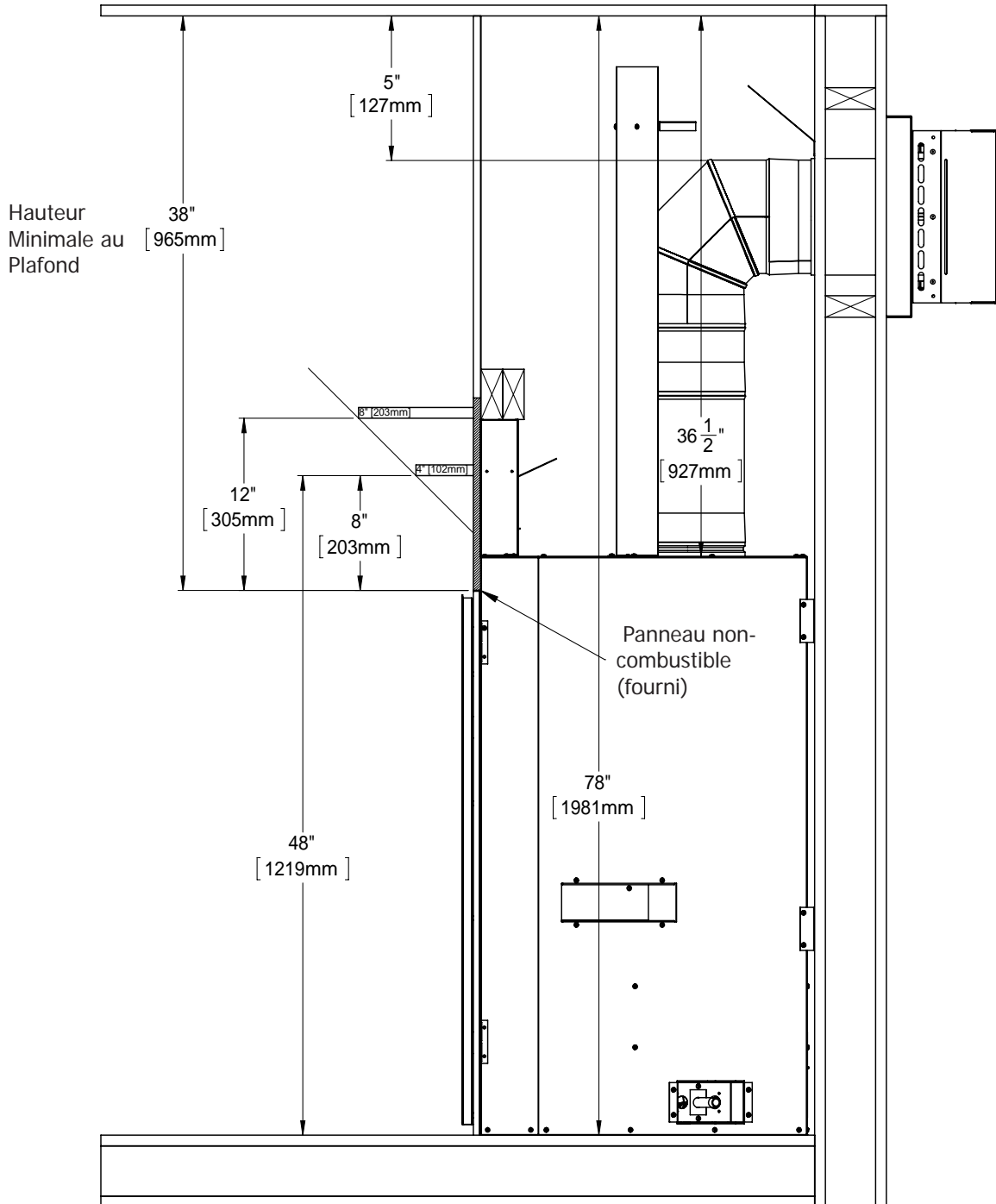
Figure 50: Installation D'un Mur Plat
