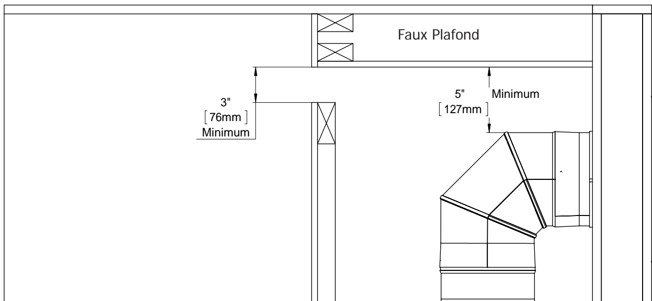
Figure 47: Faux Plafond
