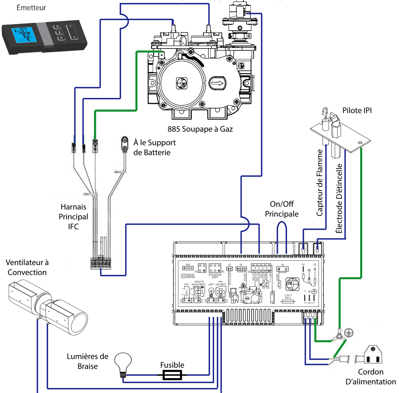
Figure 70: Diagramme de Câblage Proflame 2
