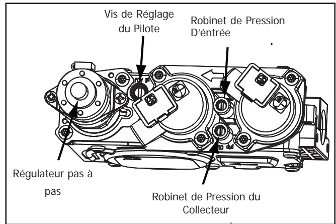
Figure 69: Vanne à Gaz Entièrement Étiquetée
