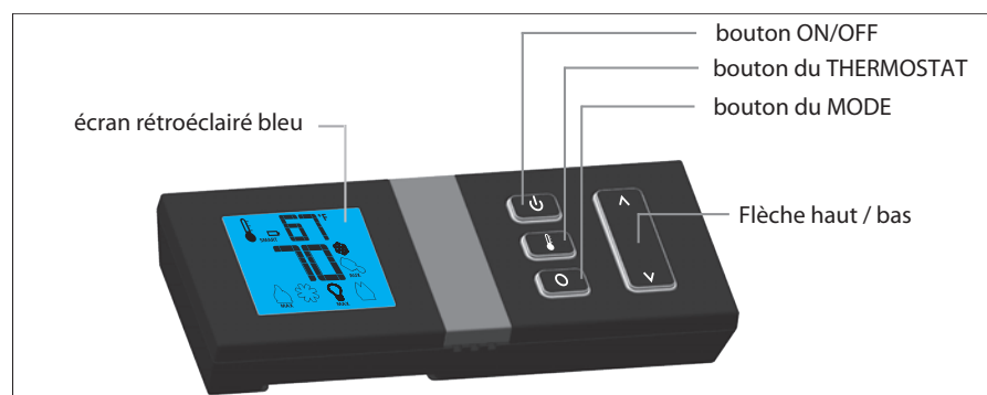
Figure 3: Émetteur Proflame 2.
