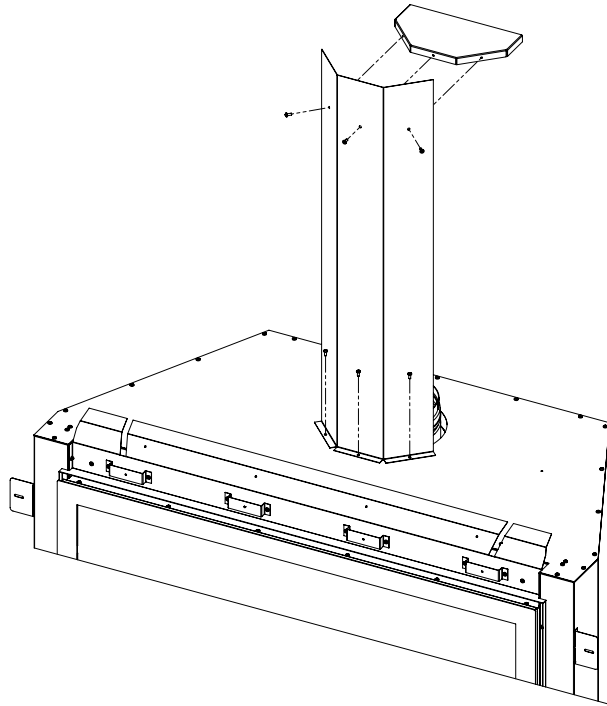
Figure 41: Boucliers D'évent
