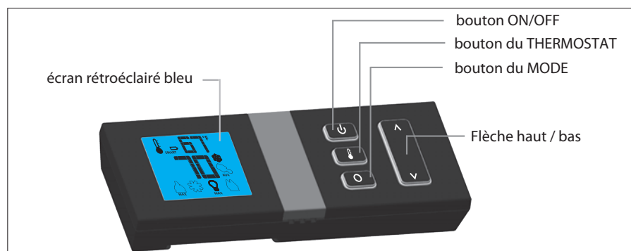
Figure 3: Émetteur Proflame 2.
