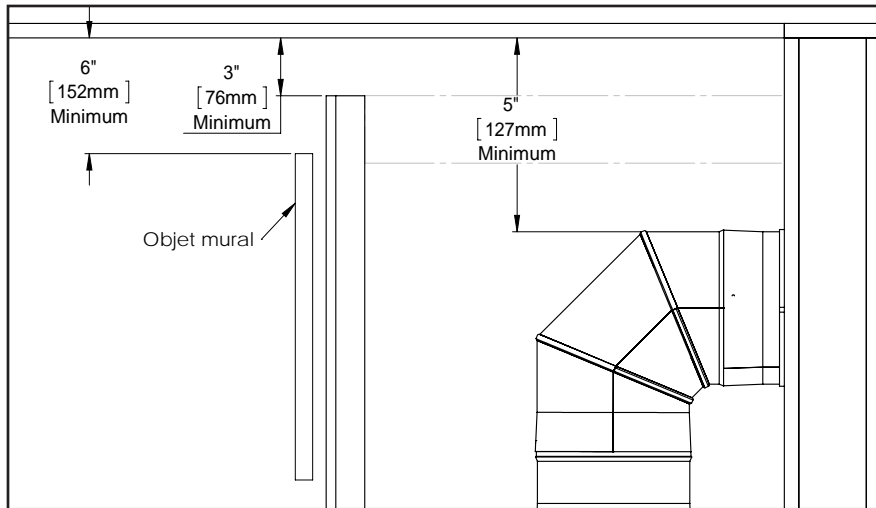
Figure 47: Option de Cadrage 2
