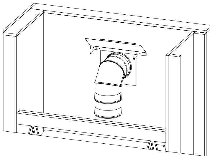
Figure 42: Bouclier Thermique Arrière
