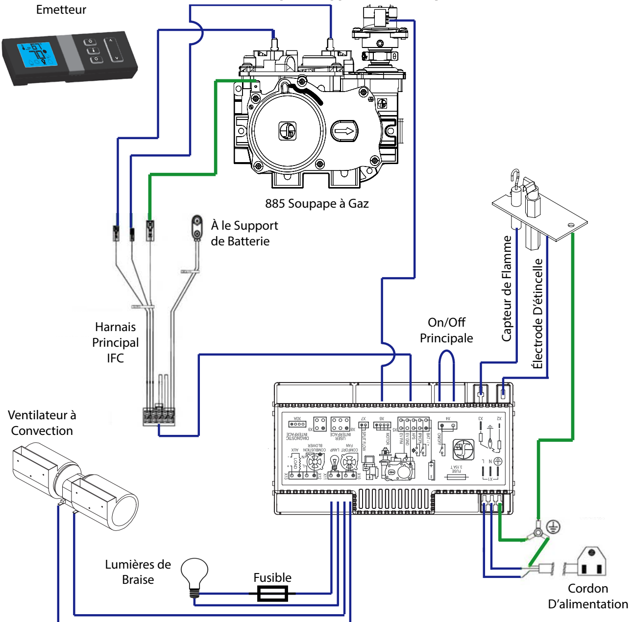
Figure 77: Diagramme de Câblage Proflame 2
