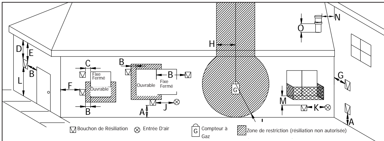
Figure 64. Restrictions de Terminaison D'évent, Référer au Tableau 3
