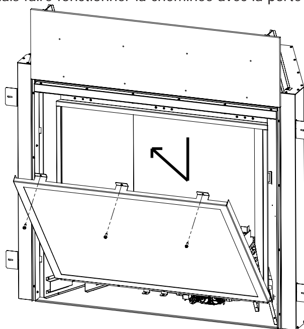
Figure 21. Enlèvement de Porte Vitrée
