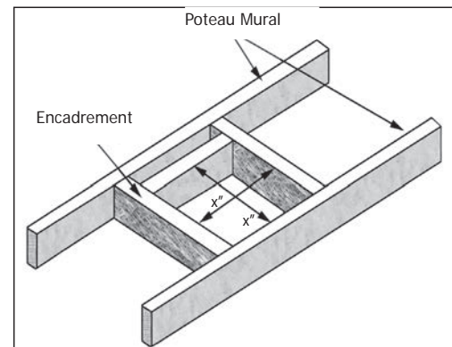
Figure 65. Encadrement dé à Coudre
