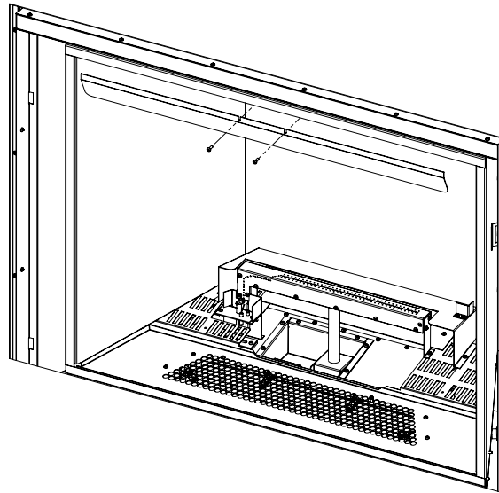
Figure 77: Enlèvement du Déflecteur de Lumière
