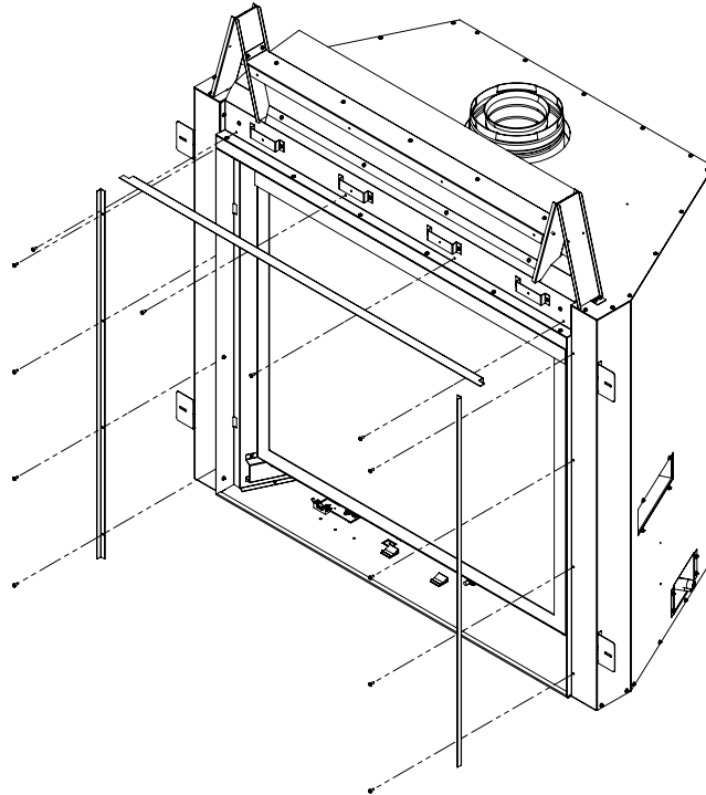
Figure 38: Installation D'Entretoise de L'Impasse
