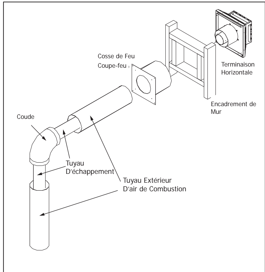
Figure 70. Terminaison de Ventilation Horizontale
