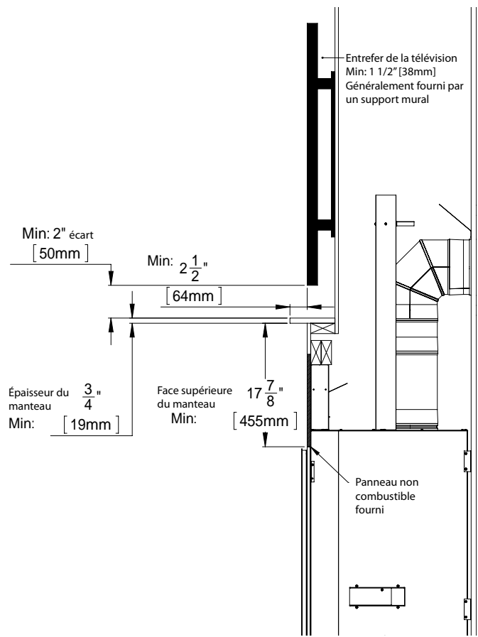
Figure 63. Installation Minimale de la Télévision Encastrée
