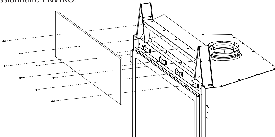
Figure 39: Installation D'Entretoise de L'Impasse
