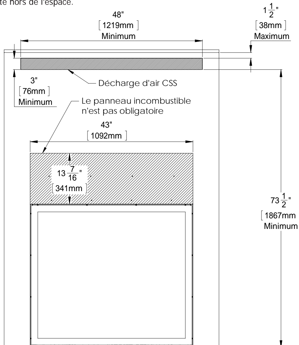
Figure 46: Option de Cadrage 1
