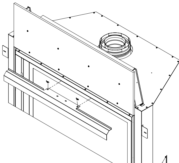
Figure 20. Enlèvement de la Couverture de Porte
