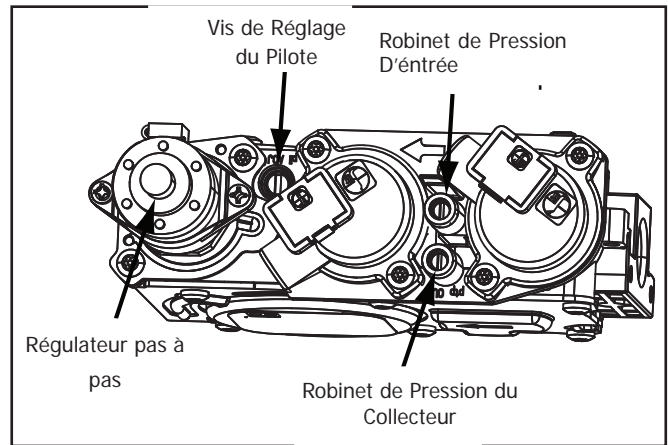
Figure 75: Vanne à Gaz Entièrement Étiquetée
