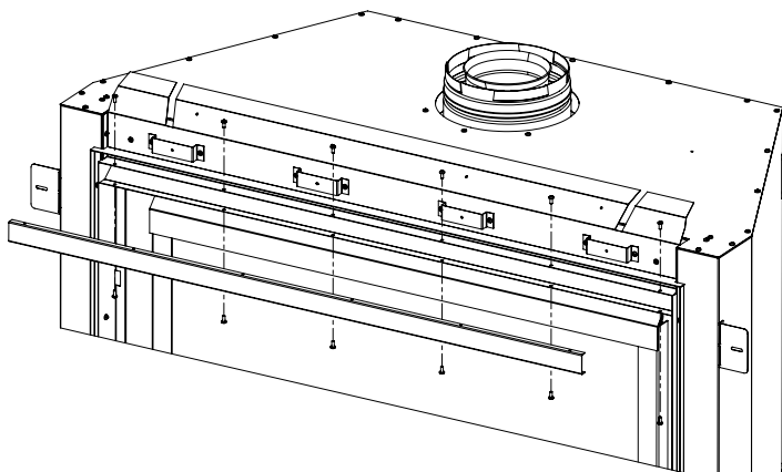
Figure 44: Retrait du capot avant
