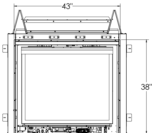
Figure 43: Dimensions du bord de finition
