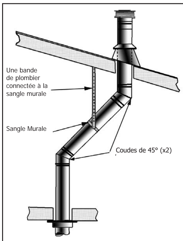
Figure 73: Installation de Tuyau D'évent Multi-Étages
