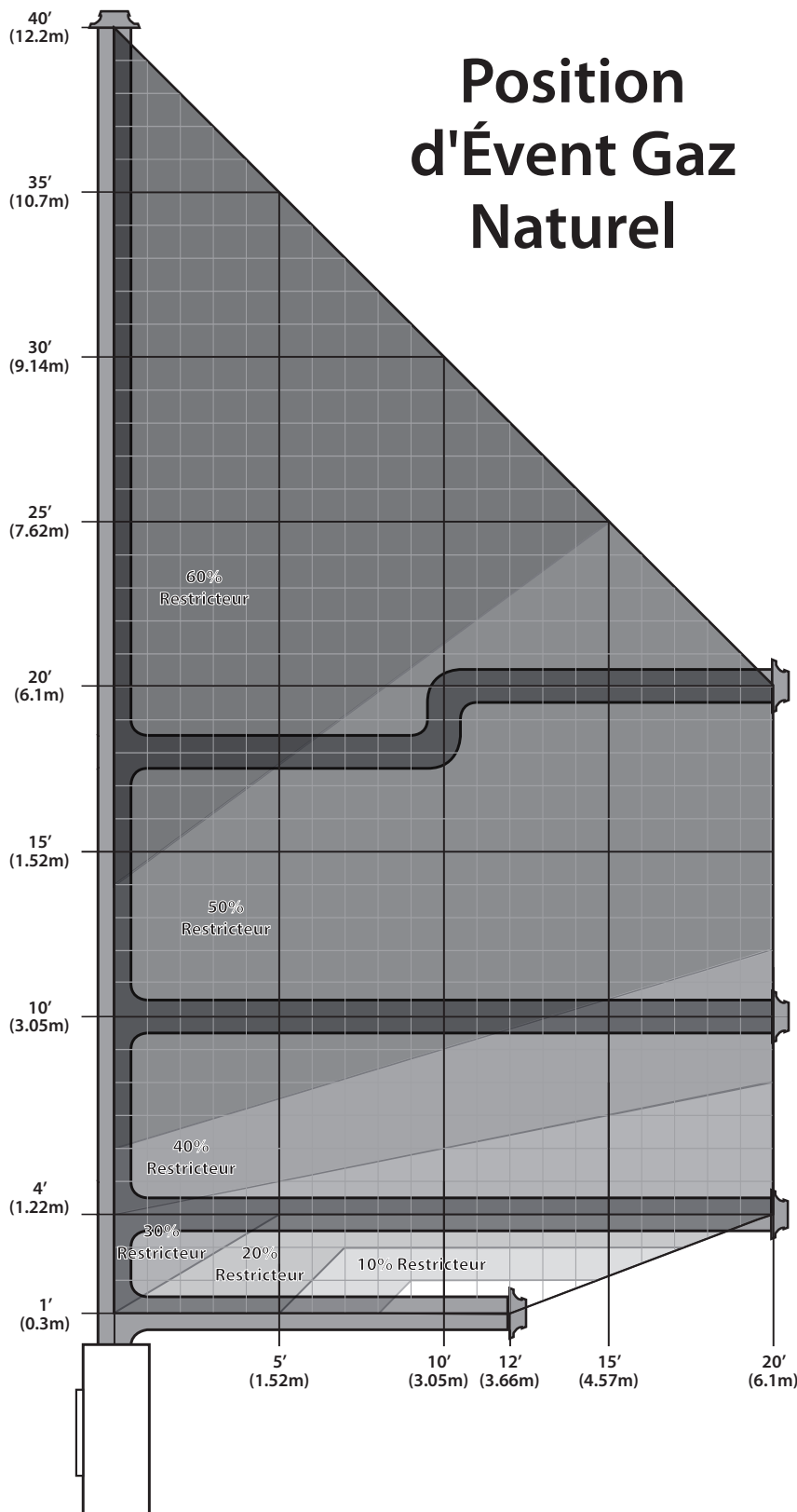
Figure 66. Graphique du Conduits Gas Naturel
