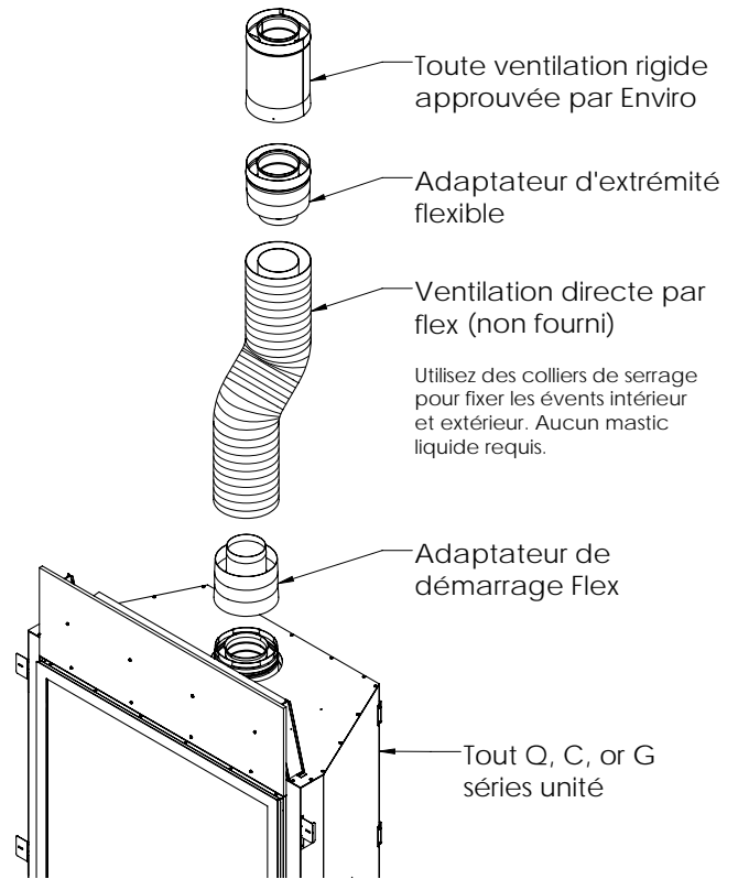
Figure 60. Installation du kit d'adaptateur Flex
