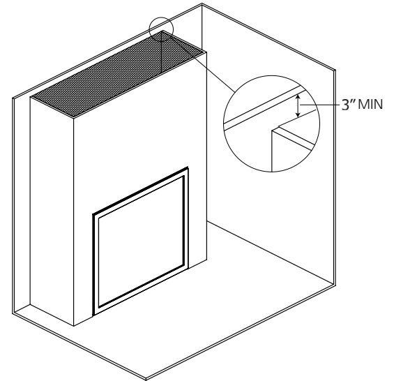
Figure 48: Vue isométrique ouverte
