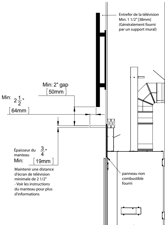
Figure 62. Installation Minimale de la Télévision
