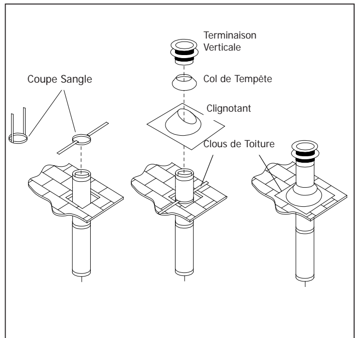
Figure 71. Terminaison Verticale de L'évent
