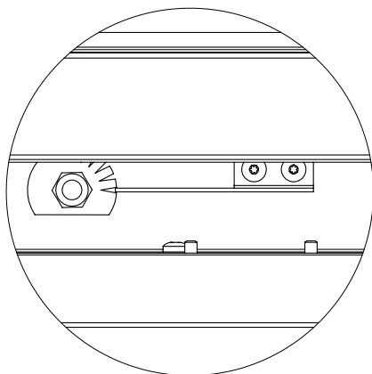
Figure 68. Réglage du Restricteur 6
