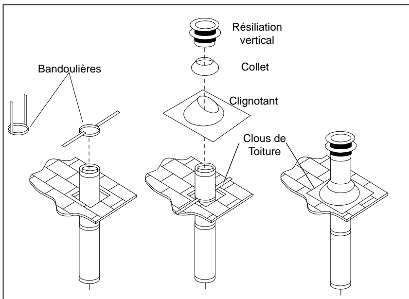
Figure 26A. Terminaison de Ventilation Verticale
