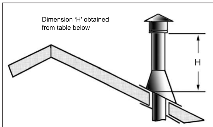
Figure 26B: Hauteur de Terminaison Verticale; Tableau de Référence 7
