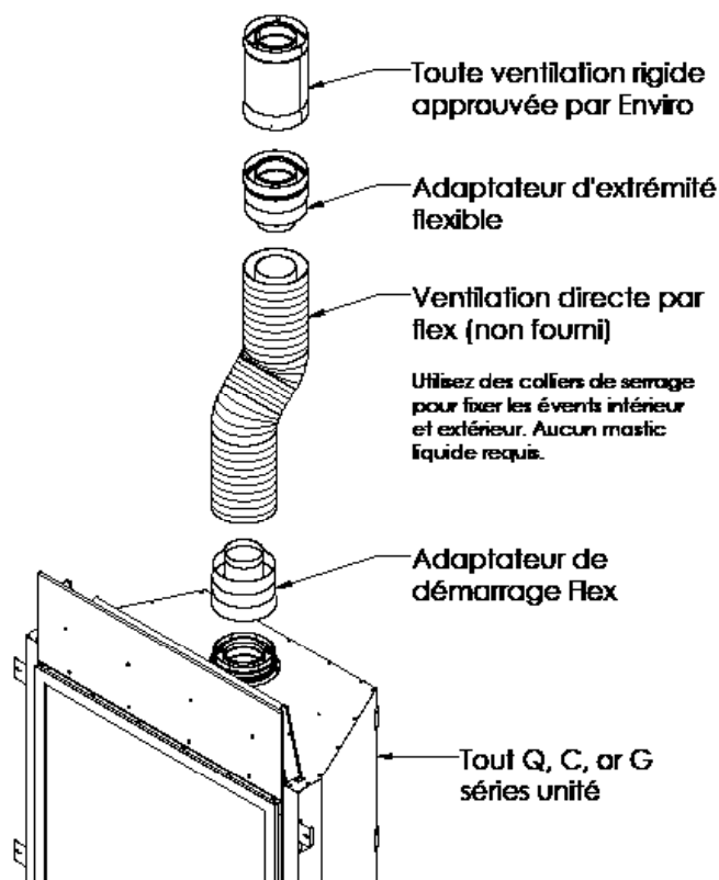
Figure 27A. Installation du kit d'adaptateur Flex
