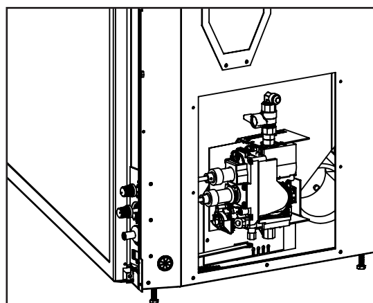
Figure 26: Tétine de tuyau mâle \frac{3}{8} " NPT avec couvercle retiré.
