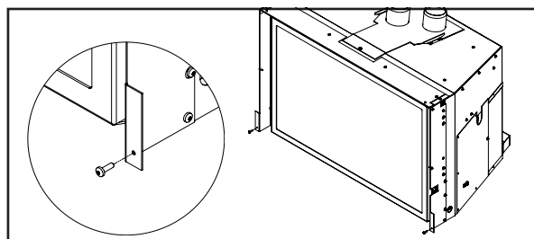
Figure 31: installation de vis à panneau réglable
