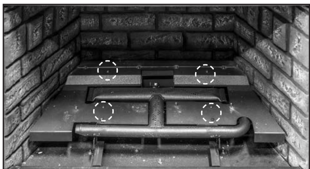
Figure 37: La grille de journal est retirée ensuite par il suffit de le soulever des languettes de montage.
