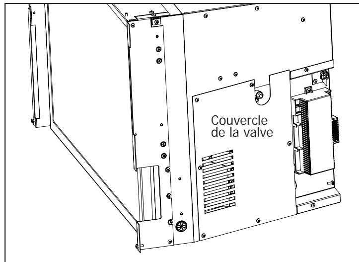
Figure 9: Couvercle de la vanne et support du brûleur.
