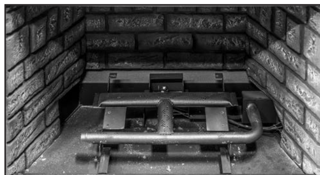
Figure 50: Retirez les 6 vis mises en évidence sur la figure 49 à l'aide d'un tournevis Torx T20 et retirez le déflecteur d'air.
