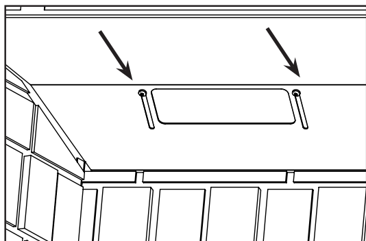
Figure 27: vis déflecteur
