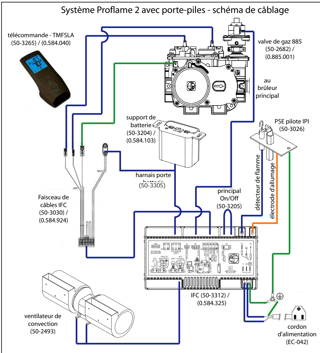
Figure 33: Schéma de Câblage
