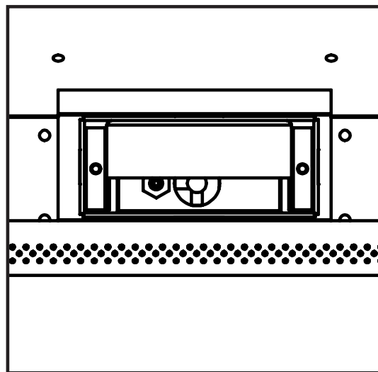
Figure 23. Ensemble d'allumage à côté du brûleur.
