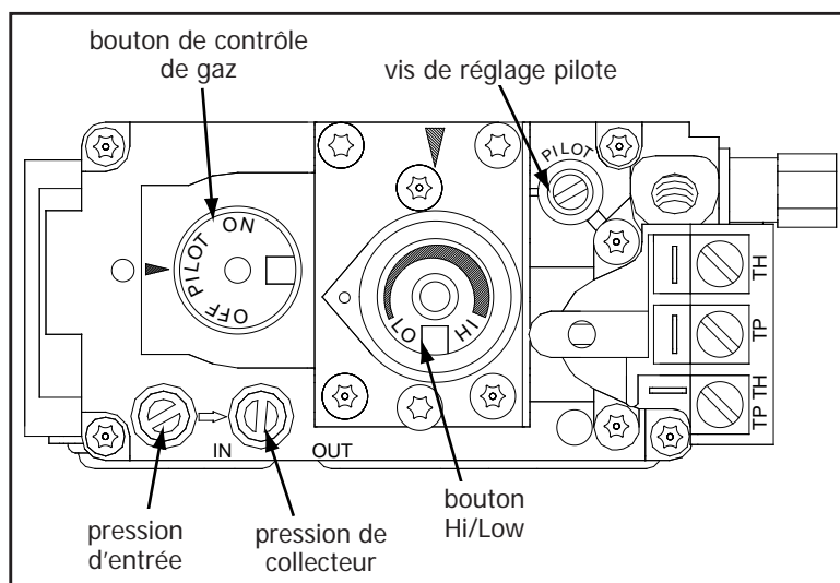
Figure 27: Détails de la valve.
