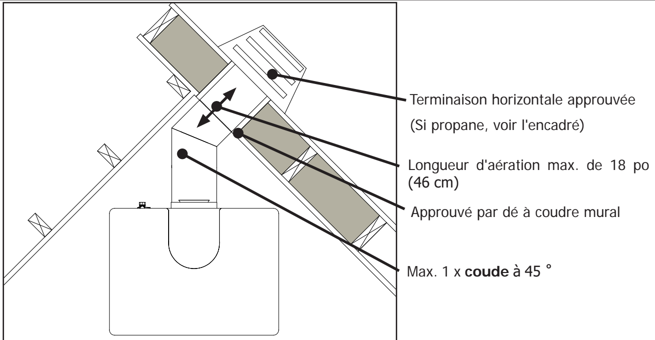
Figure 32: Événement d'angle arrière - Pas d'élévation verticale
