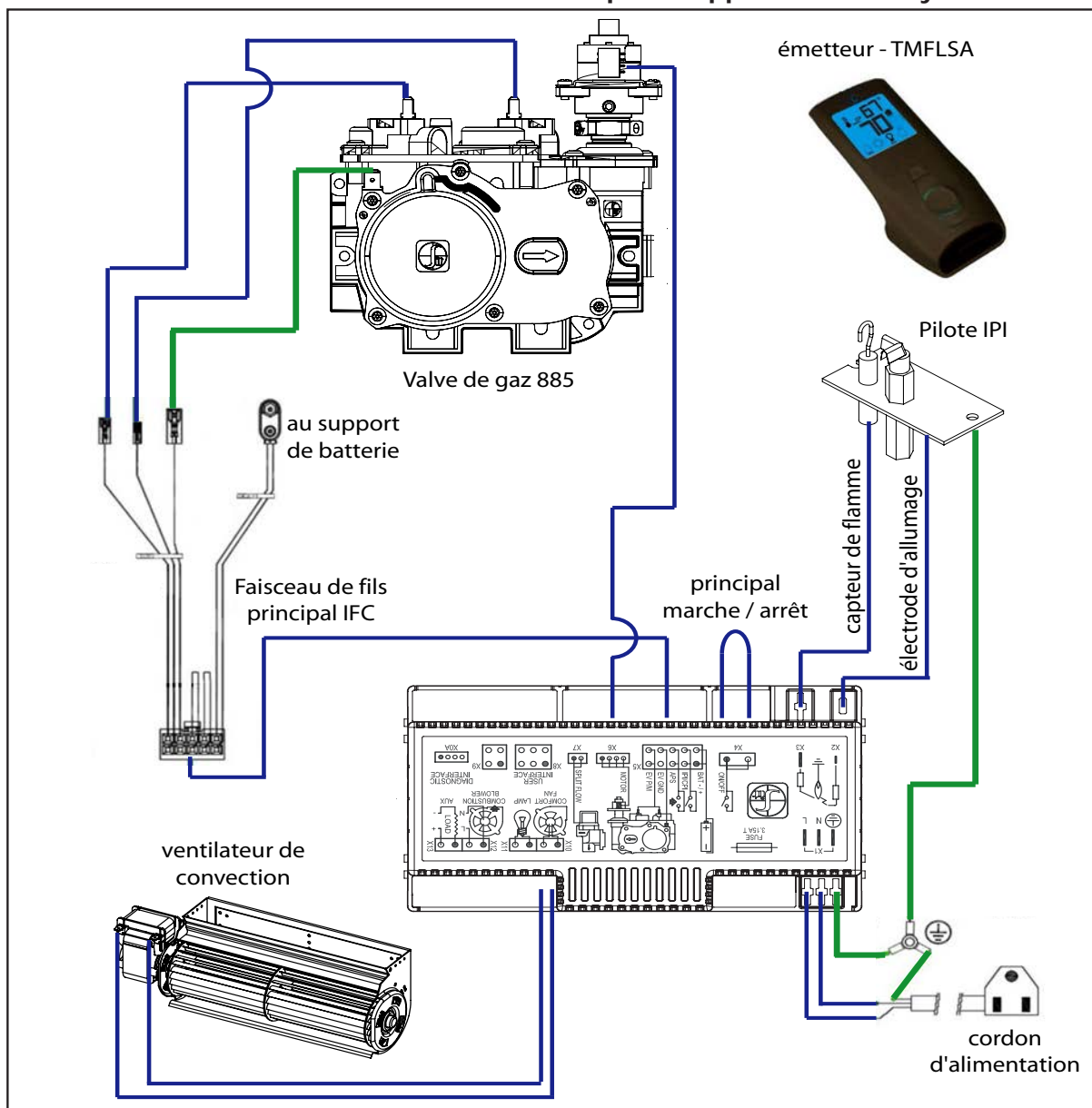
Figure 44: Schéma de câblage
