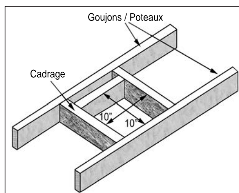
Figure 31: Encadrement de dé à coudre d'aération
