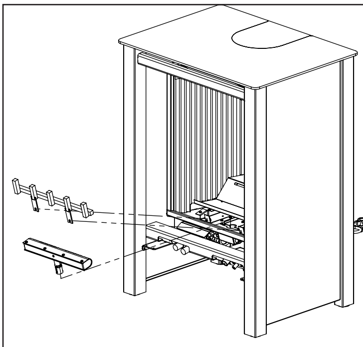
Figure 20: Retrait du brûleur
