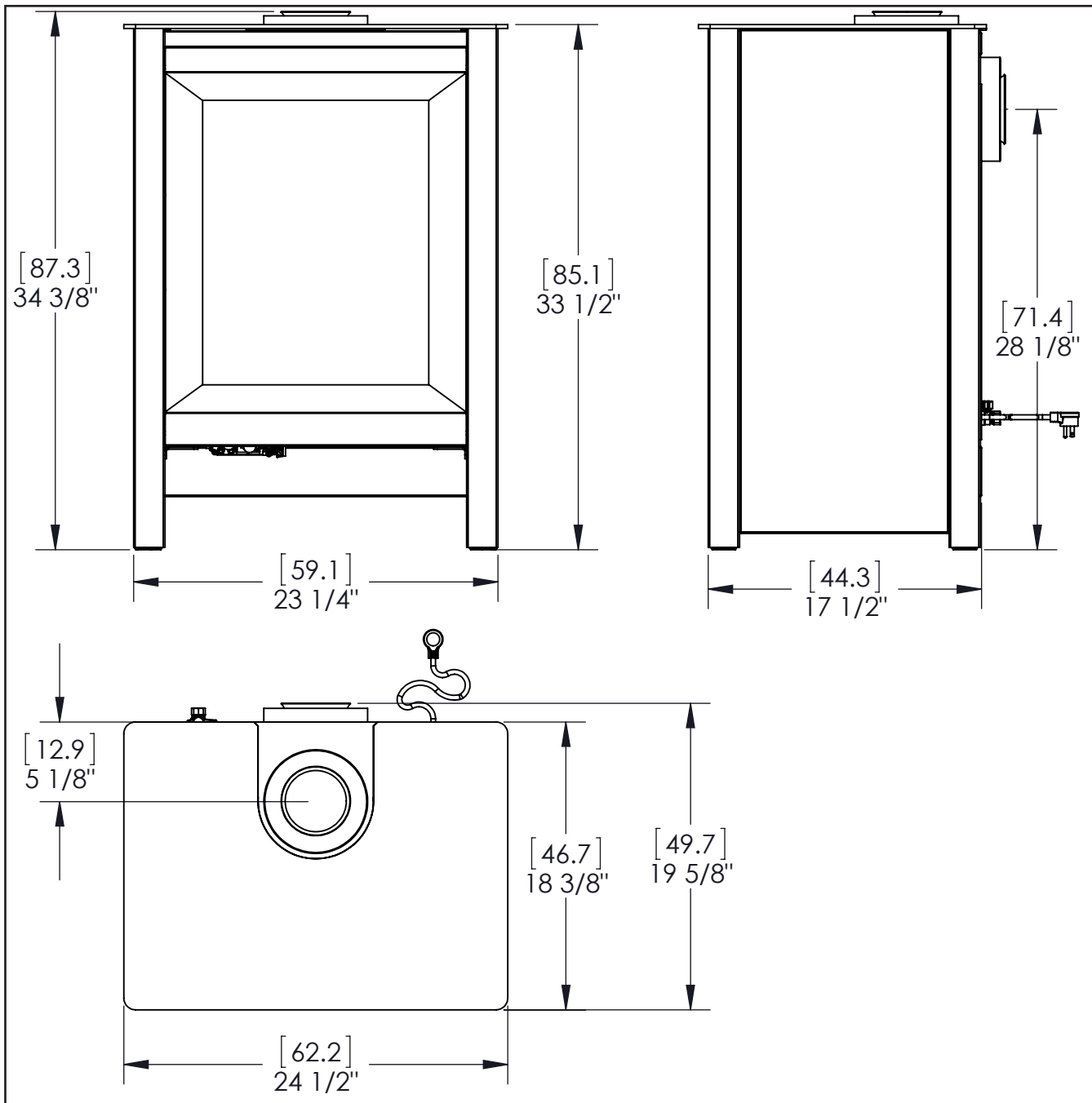
Figure 1: Dimensions S201/S201D - Évén supérieur
