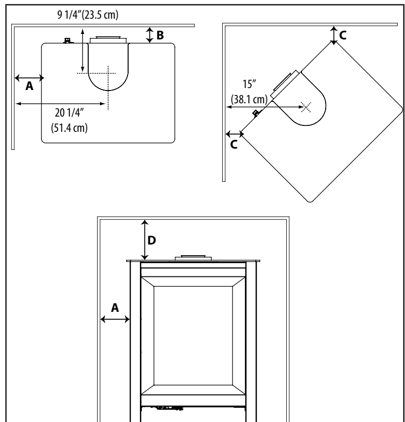
Figure 24: Dégagement des combustibles
