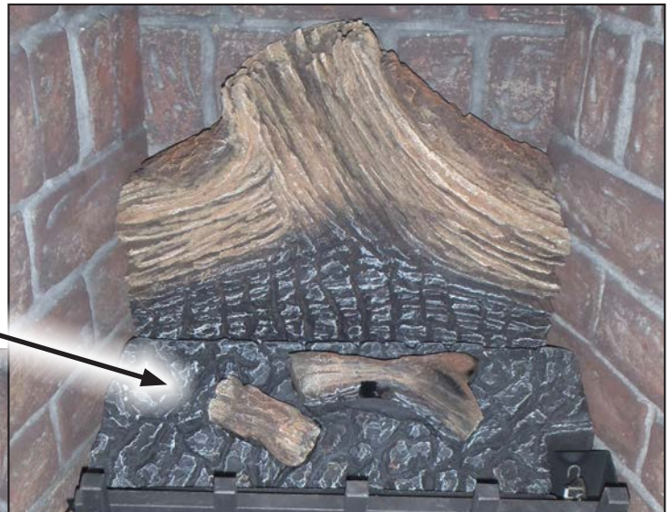
Figure 46: Installation de bûches arrière et de lit de braises.
