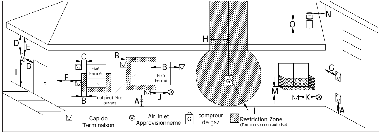
Figure 30: Restrictions relatives à la terminaison de l'évent, voir le tableau 2
