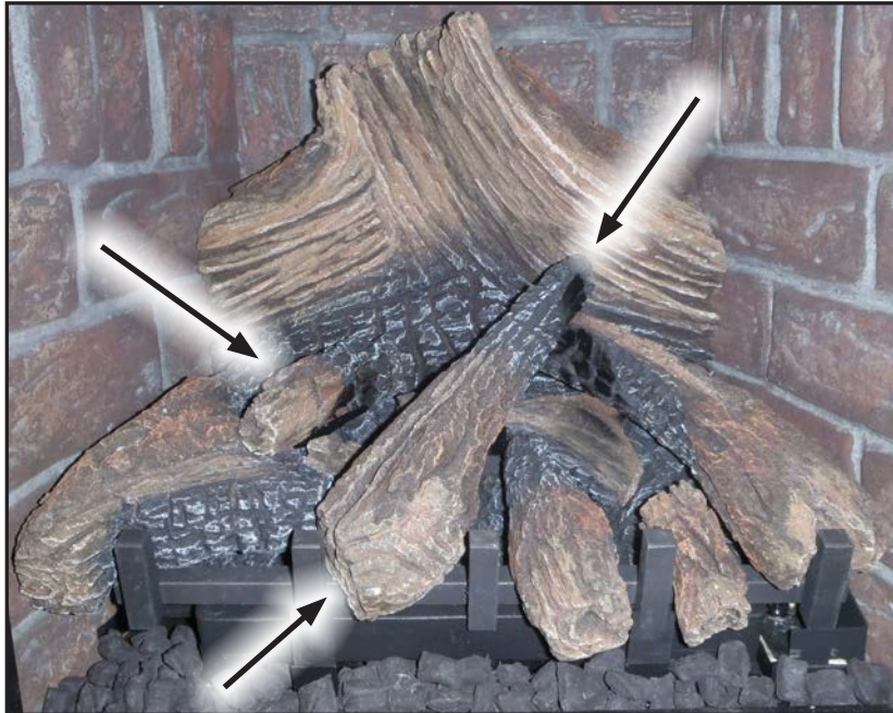
Figure 50: Installation complète de bûches avec braises.
