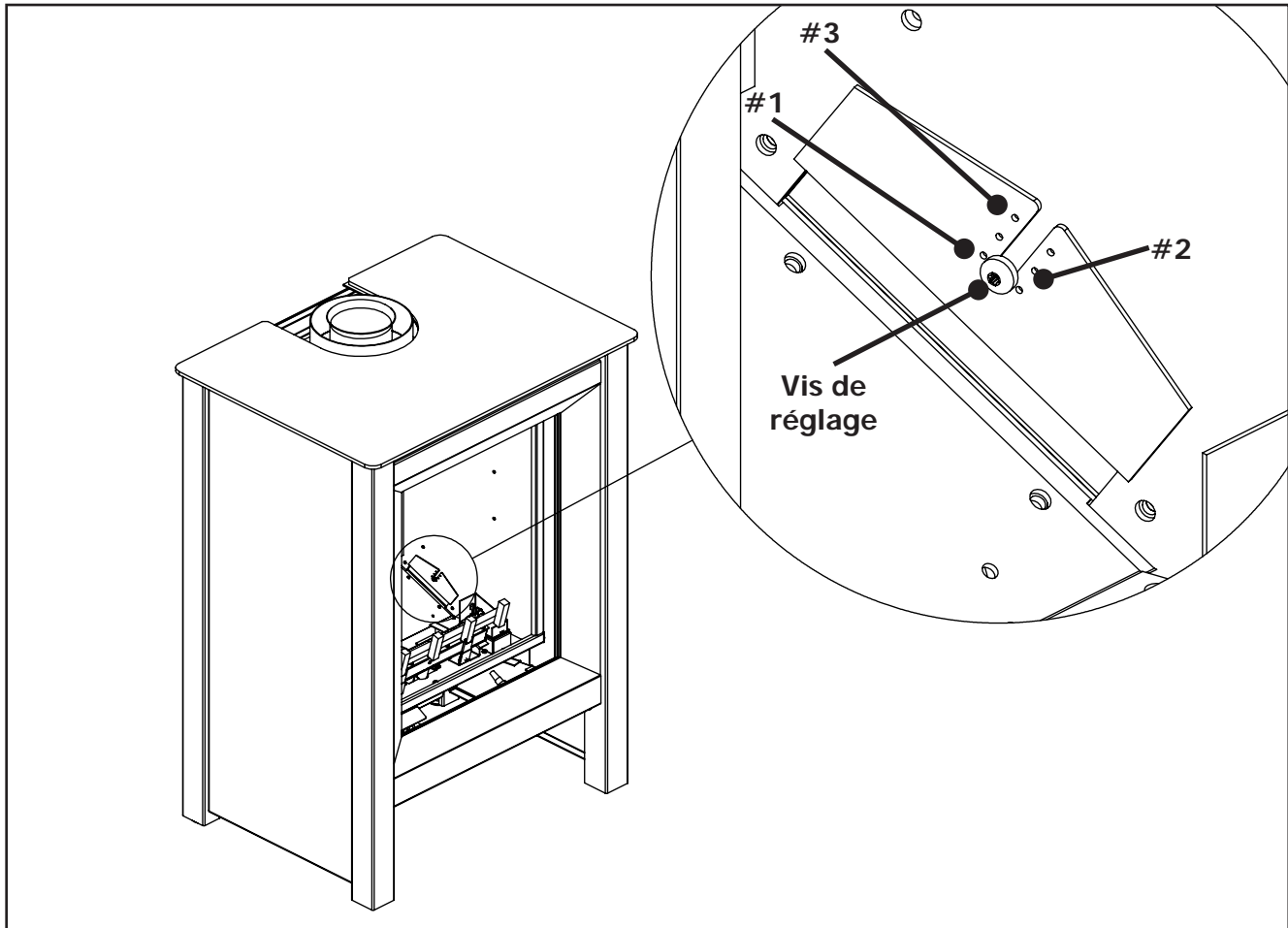
Figure 42: Installation de restricteurs d'air
