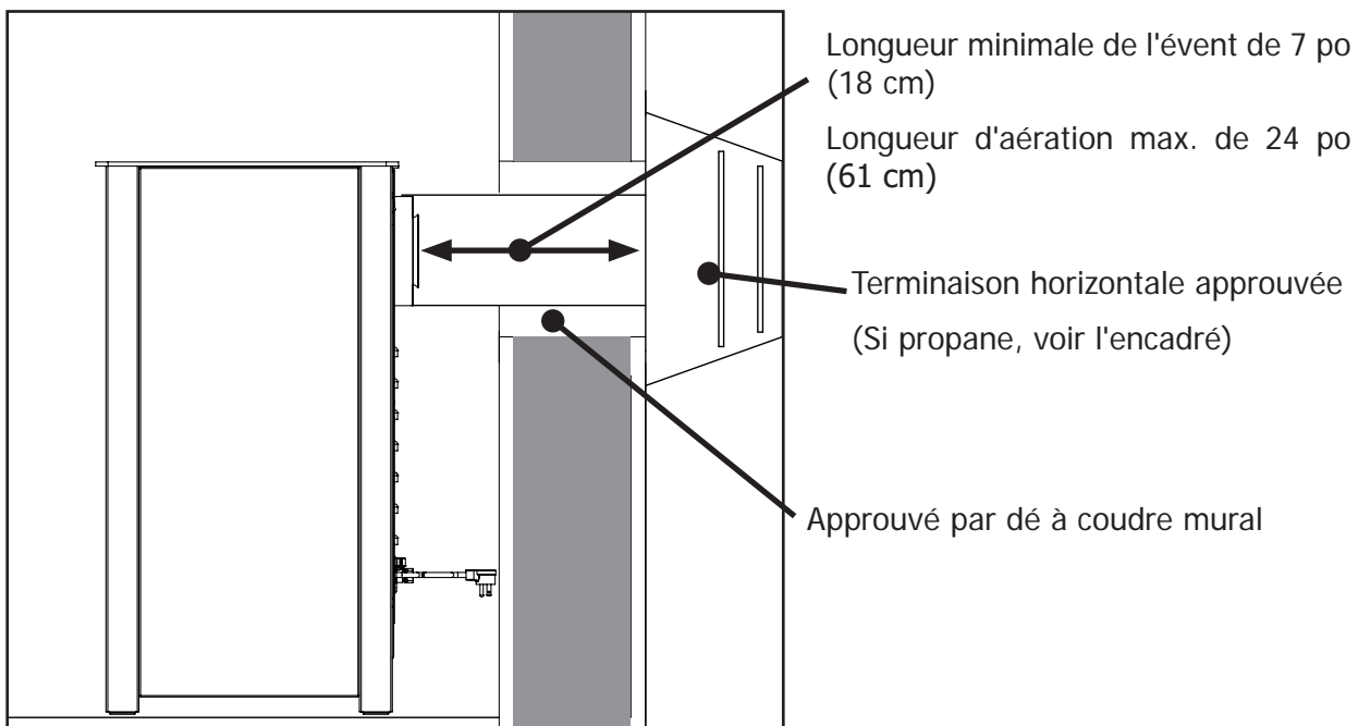
Figure 33: Événement arrière à paroi plate - Aucune élévation verticale
