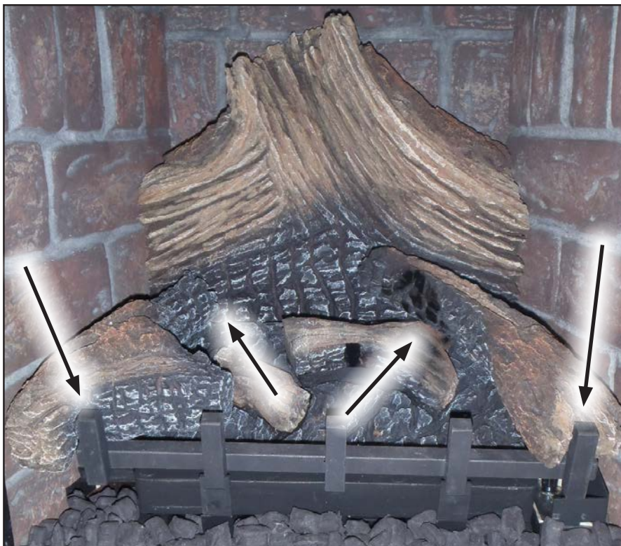
Figure 48: Installation de l'ensemble de bûches de troisième étape.
