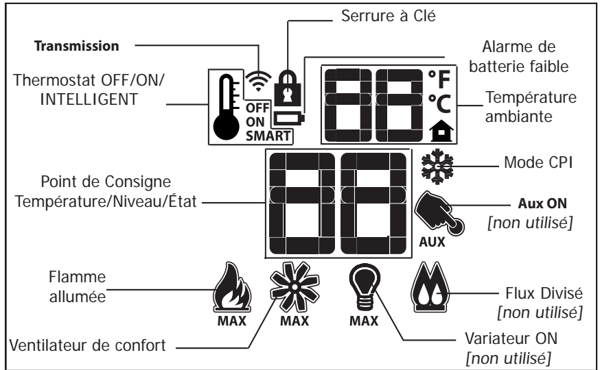
Figure 5: Écran LCD de l'émetteur Proflame 2.
