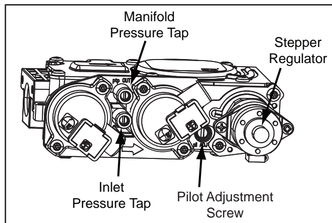
Figure 43: Vanne à gaz entièrement étiquetée Consultez le manuel d'utilisation de Dexen pour plus de détails sur la vanne S201D
