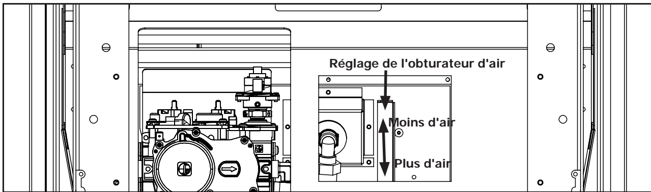
Figure 3: Levier d'obturation d'air
