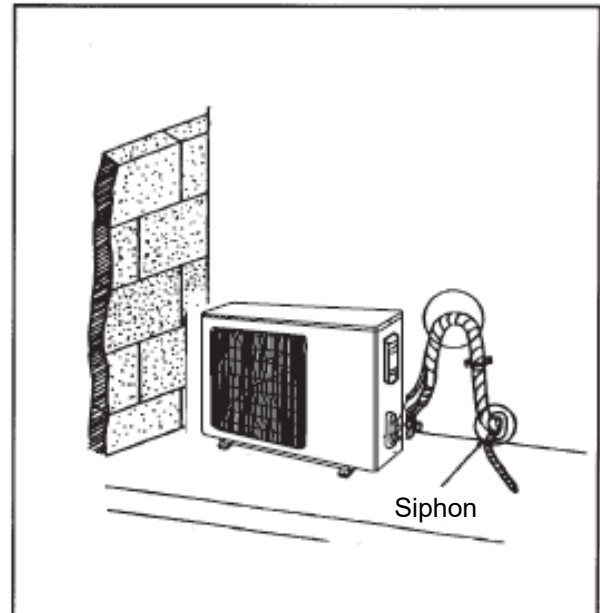
L'unité extérieure installée plus haut que l'unité intérieure
