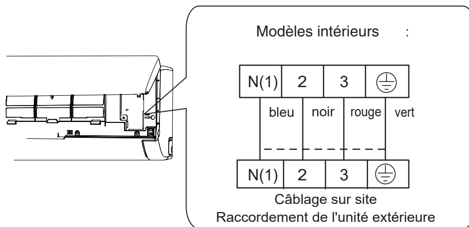
Exemple de câblage intérieur
