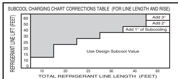
1 1/2 Ton Heat Pump
