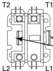
Contacteur unipolaire (MS)*
