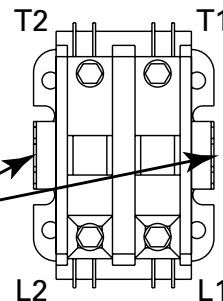
Contacteur bipolaire (MS)*
